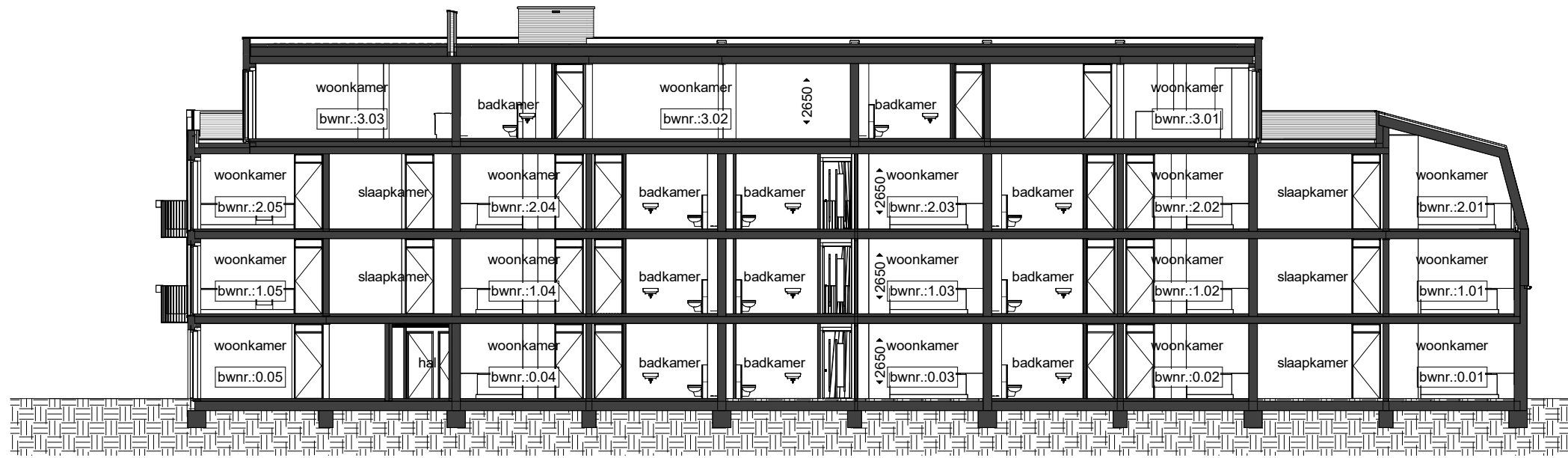
Doorsnede A VK
