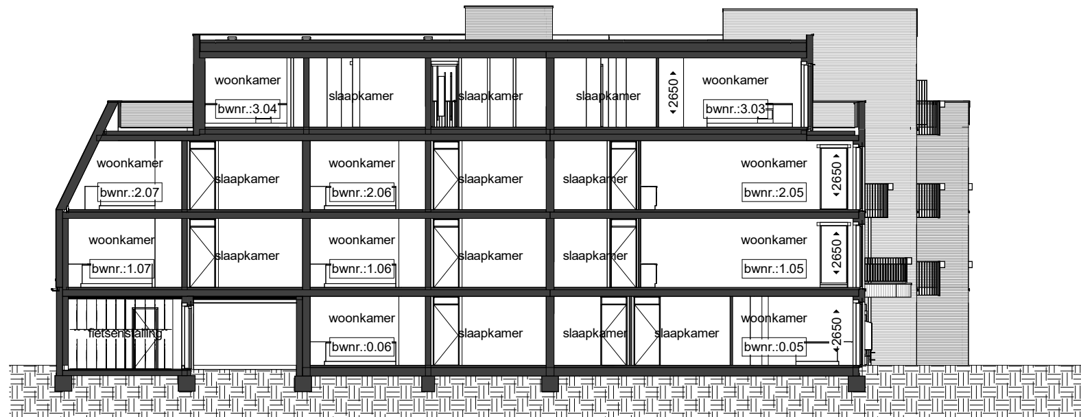
Doorsnede B VK
