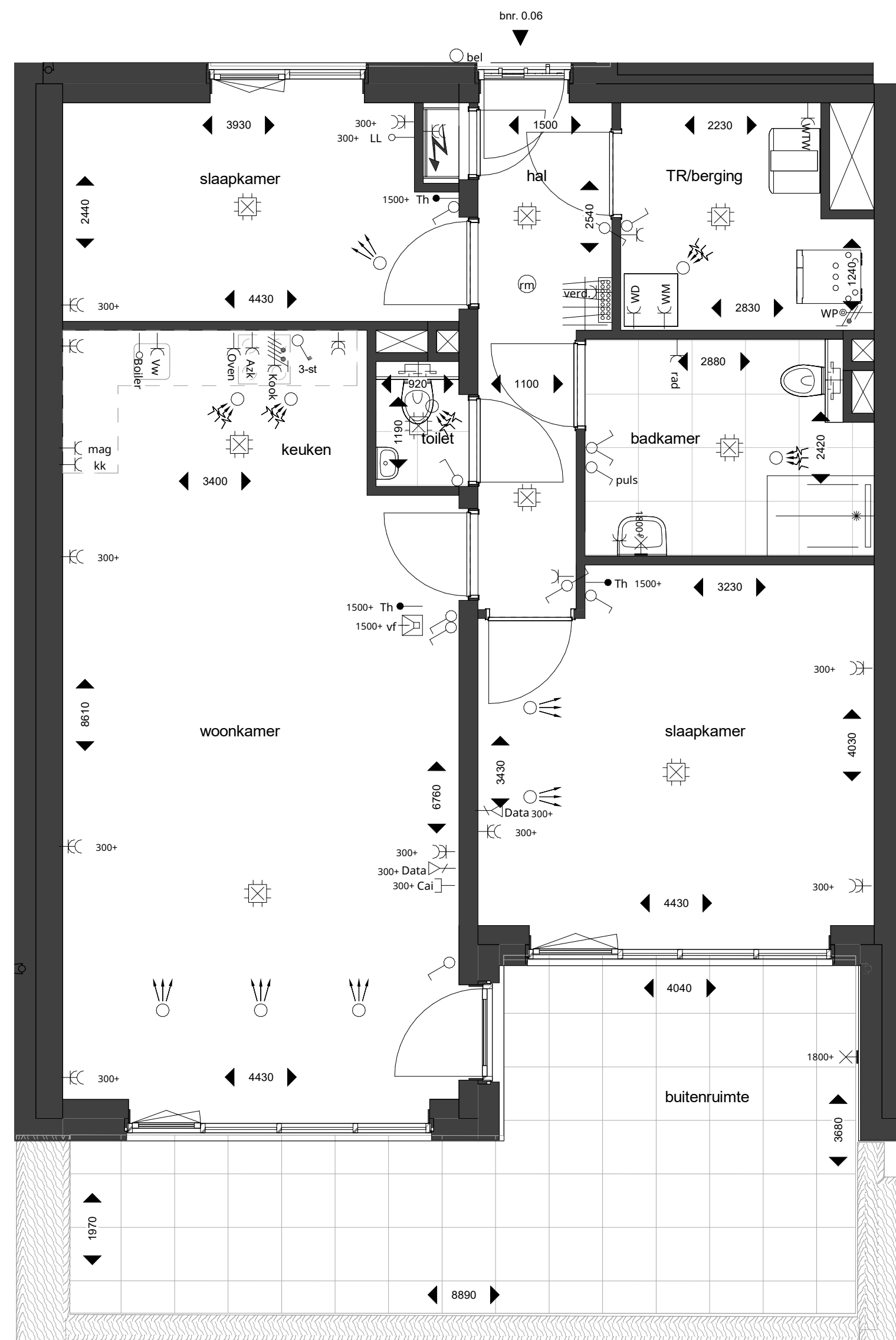
plattegrond bnr. 0.06
