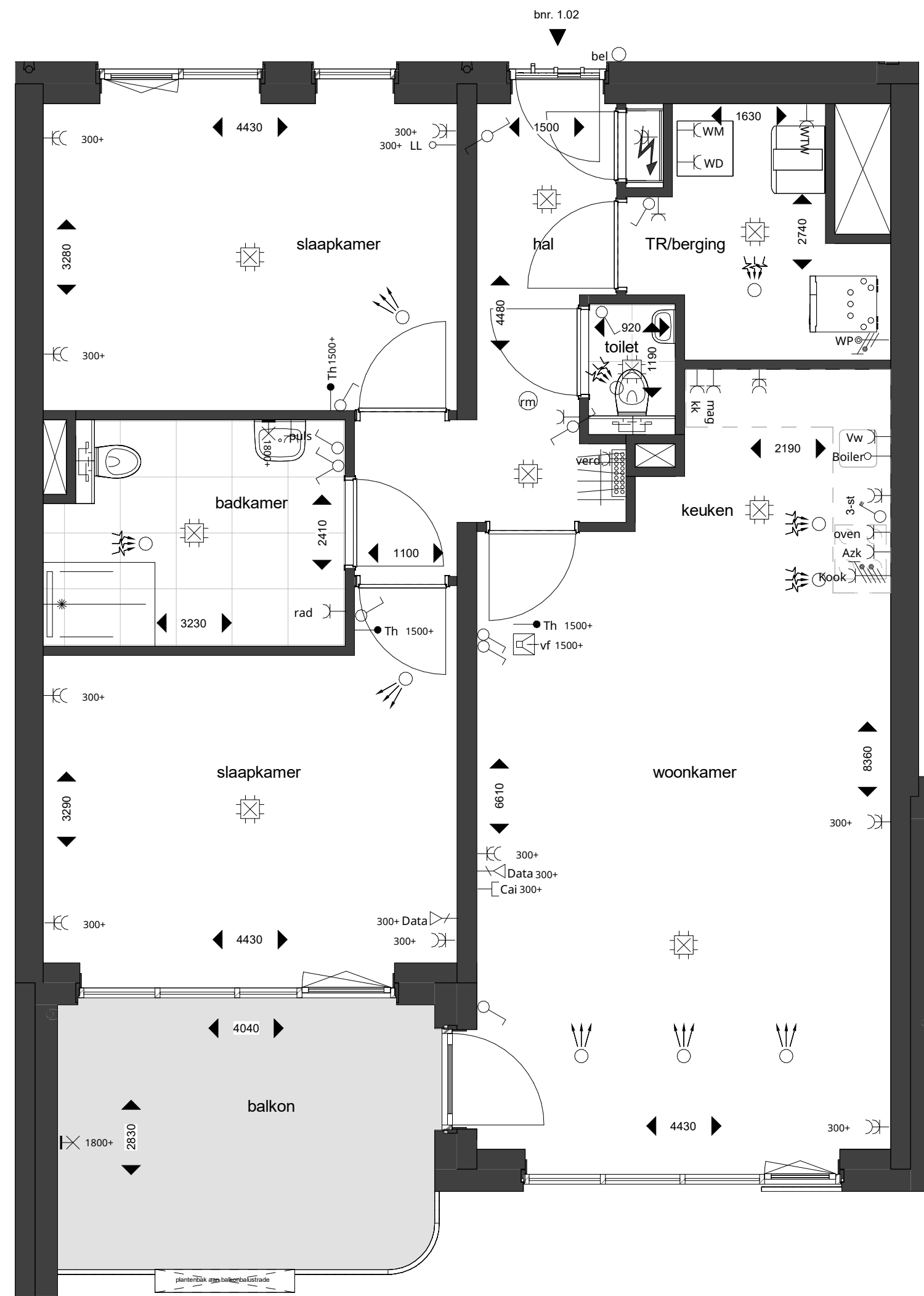
plattegrond bnr. 1.02
