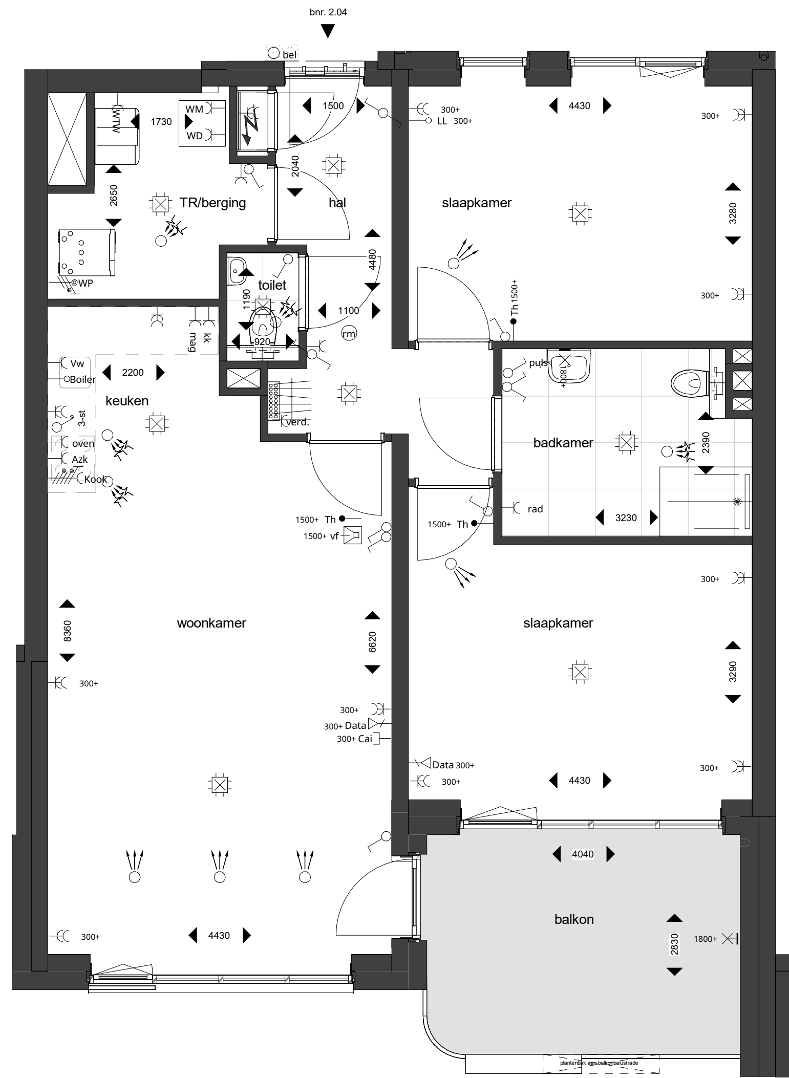
plattegrond bnr. 2.04
